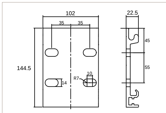
SUPPORT POSE FACE ET PLAFOND
