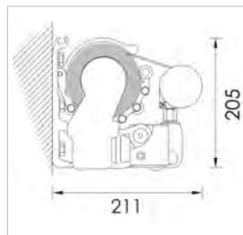
POSE DE FACE AVEC AUVENT BRAS RENFORCE
