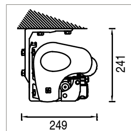
POSE PLAFOND
