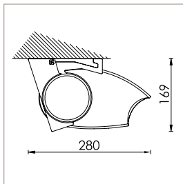
POSE PLAFOND AVEC INCLINAISON 85°
