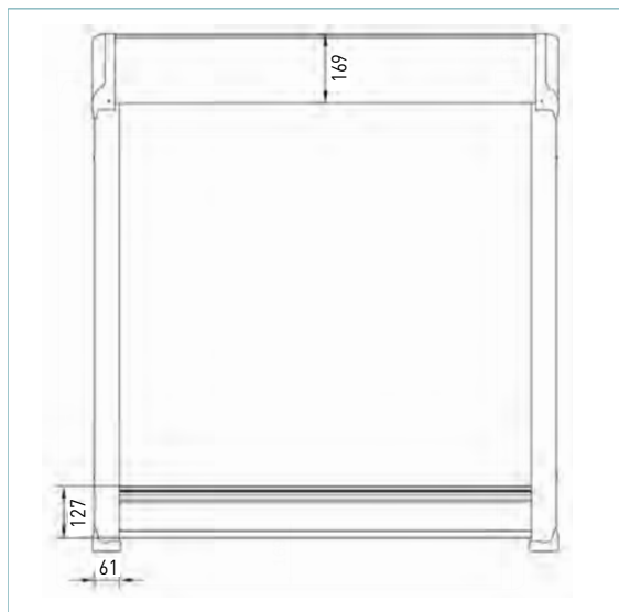
POSE SUR EQUERRES
