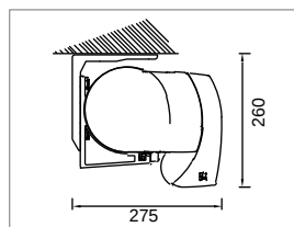
POSE PLAFOND AVEC LAMBREQUIN DÉROULABLE
