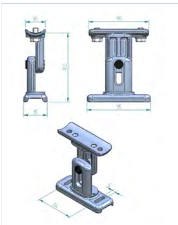
FIXATIONS AU SOL
