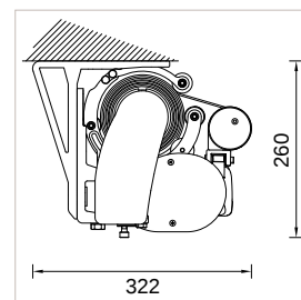
POSE PLAFOND AVEC INCLINAISON 45°
