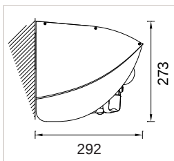
POSE DE FACE AVEC AUVENT
