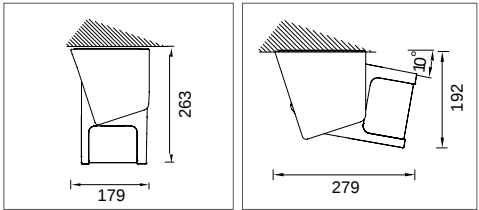
POSE PLAFOND
