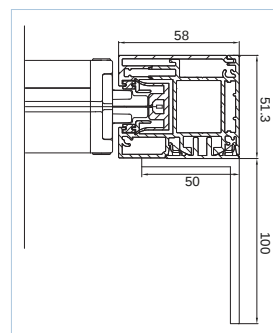
COULISSE AVEC EQUERRE
