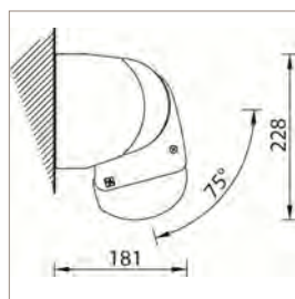
POSE FACE AVEC INCLINAISON 75°
