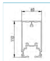
SECTION DES GUIDES
