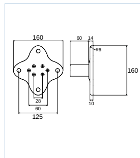
FIXATION COLONNE
