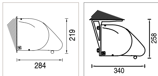
AVEC LAMBREQUIN DEROULABLE
