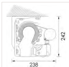
POSE DE FACE AVEC AUVENT
