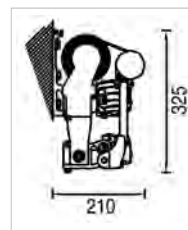
BRAS CROISÉS
