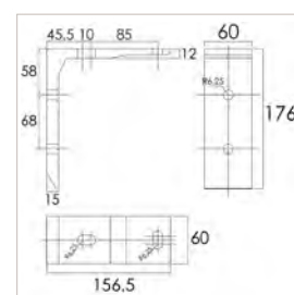
EQUERRE POSE PLAFOND
