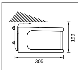
POSE PLAFOND
