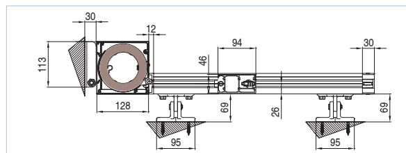
COFFRE CARRÉ - 130
