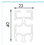
SECTION DES TRAVERSES
