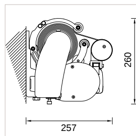
POSE DE FACE AVEC INCLINAISON 45°
