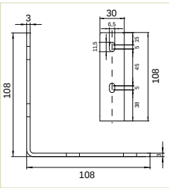
EQUERRE POSE LATÉRALE
