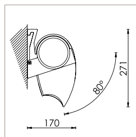
POSE FACE AVEC INCLINAISON 80°
