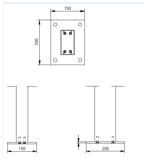
FIXATIONS AU SOL
