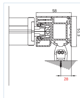
COULISSE AVEC SUPPORT POSE A PLAT
