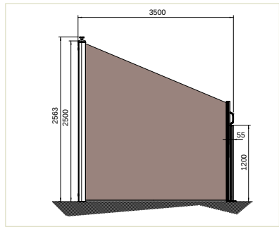
EQUERRE POSE LATÉRALE
