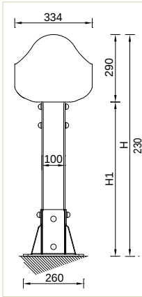
VUE LATÉRALE
