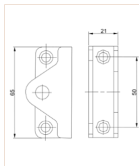
FIXATION DU BRAS
