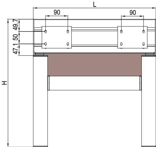
Vue arrière
