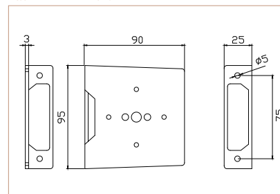
EQUERRE DE FIXATION
