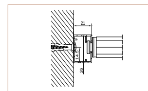
COULISSE POSE TABLEAU
