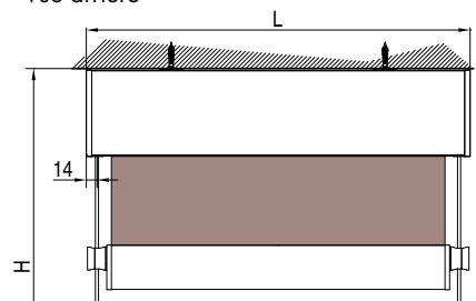
Vue arrière
