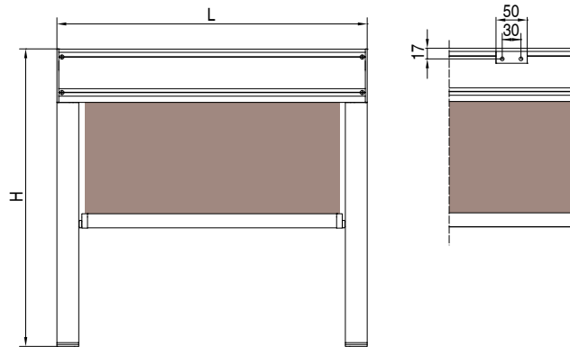
Vue arrière
