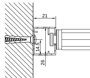
Coulisse pose tableau
