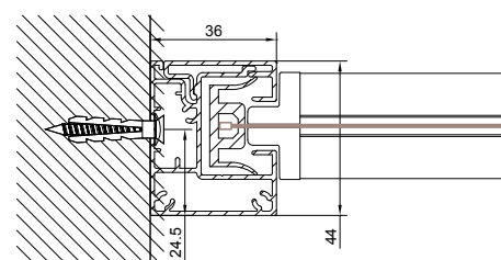
Coulisse pose tableau
