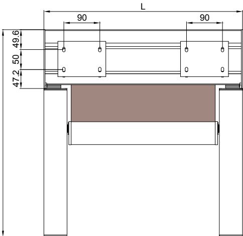
Vue arrière
