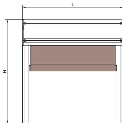
Vue arrière
