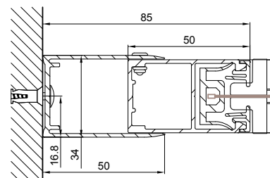
Coulisse pose tableau
