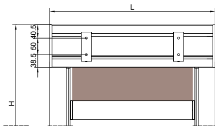
Vue arrière
