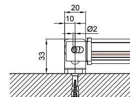
Support pour équerre inférieure pose face
