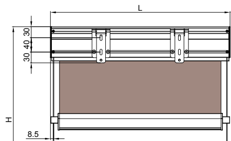
Vue arrière
