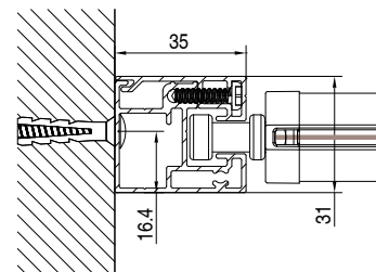
Coulisse pose tableau
