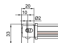
Équerre inférieure pose tablette
