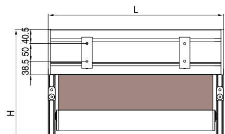
Vue arrière
