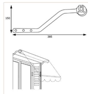
SUPPORT PERSIENNE +101€ la paire
