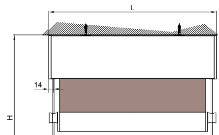
Vue arrière
