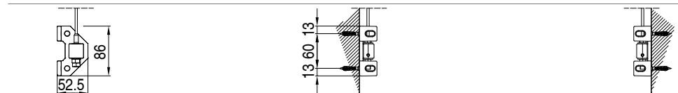
Équerre inférieure pose tablette
