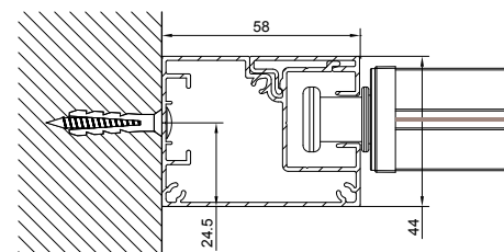
Coulisse pose tableau
