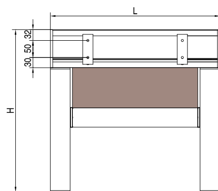
Vue arrière
