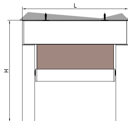
Vue arrière
