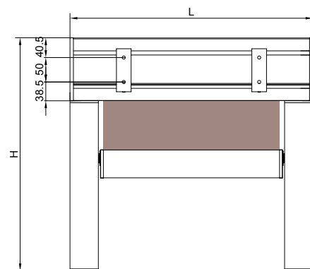
Vue arrière
