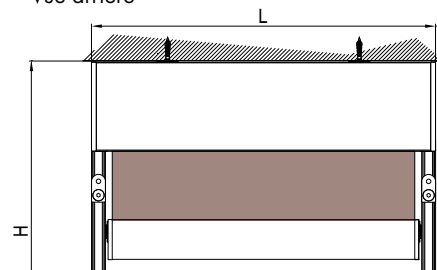
Vue arrière
