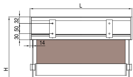
Vue arrière
